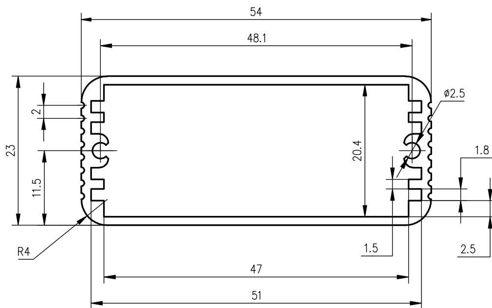
Профиль BIS-S1
